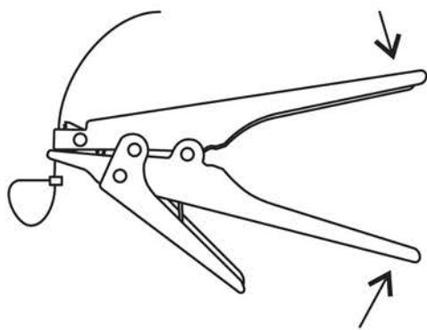
Рисунок 3 – Затяжка кабельного хомута с помощью ПКХ-519
