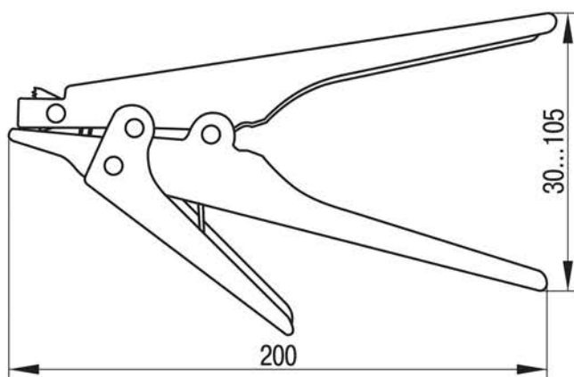
Рисунок 1 – ПКХ-519
