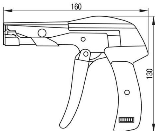
Рисунок 2 – ПКХ-600А
