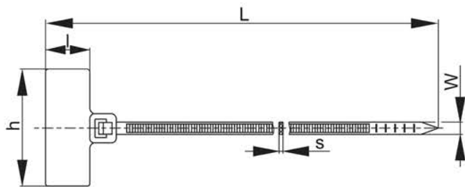
а) хомут типа ХП1
