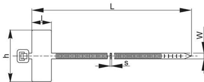
б) хомут типа ХП2
