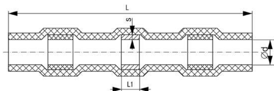
Рисунок 3 – Гильза ГСИ-п
