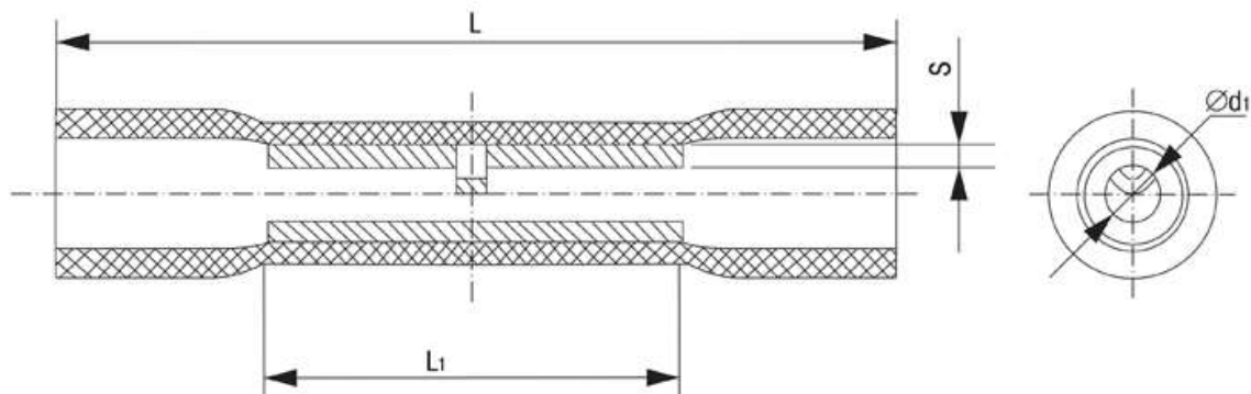
Рисунок 2 – Гильза ГСИ-т
