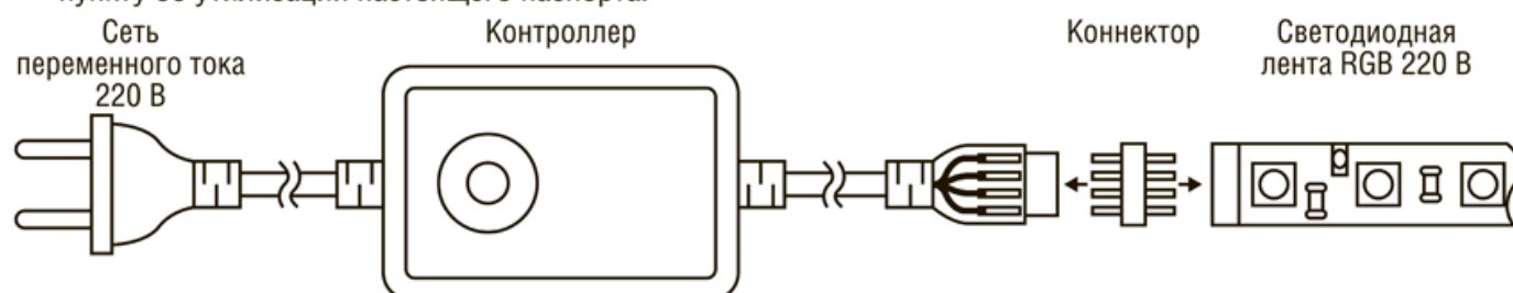
Рис. 2. Подключение
