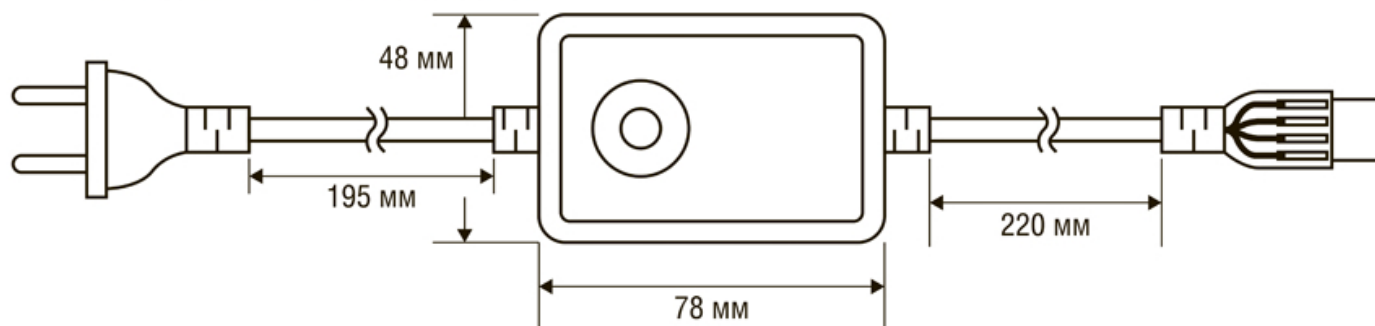
Рис. 1. Габаритные и установочные размеры контроллера.
