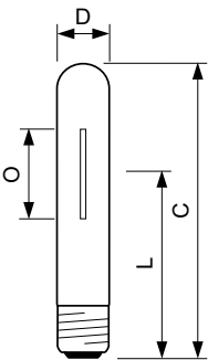
SON-T APIA Plus Xtra 150W E40
