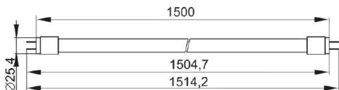
Рисунок 29 – Лампа LED–T8, 10 Вт, 13 Вт, цоколь G13
