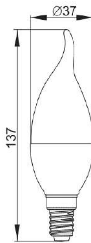
Рисунок 8 – Лампа LED-CB35, 5 Вт, 7 Вт, цоколь E14
