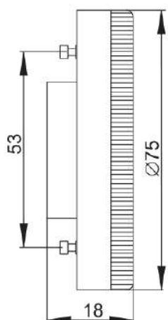
Рисунок 25 – Лампа LED–T75, 10 Вт, цоколь GX53
