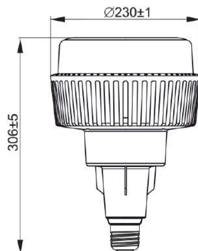
Рисунок 38 – Лампа LED- HP, 160 Вт, цоколь E40
