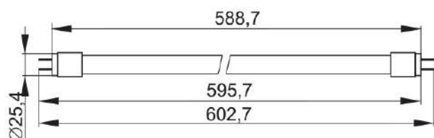
Рисунок 29 – Лампа LED–T8, 10 Вт, 13 Вт, цоколь G13
