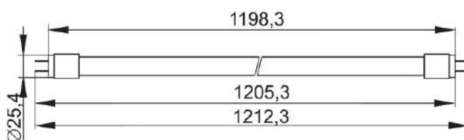
Рисунок 30 – Лампа LED–T8, 18 Вт, 20 Вт, 25 Вт, 30 Вт, 40 Вт, цоколь G13
