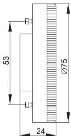
Рисунок 26 – Лампа LED–T75, 12 Вт, цоколь GX53
