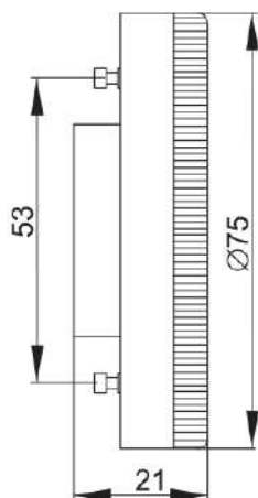
Рисунок 27 – Лампа LED–T75, 15 Вт цоколь GX53
