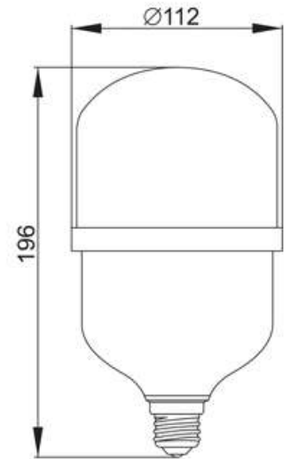
Рисунок 28 – Лампа LED– HP, 30 Вт, цоколь E27
