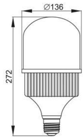
Рисунок 35 – Лампа LED-HP, 80 Вт, 100 Вт, цоколь E40
