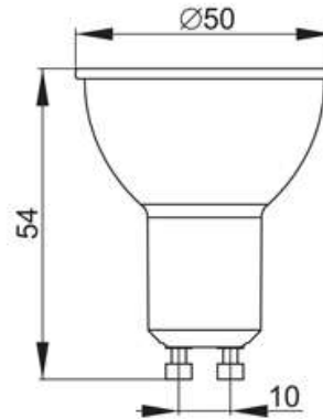
Рисунок 19 – Лампа LED–PAR16, 5 Вт цоколь GU10
