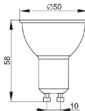
Рисунок 20 – Лампа LED–PAR16, 7 Вт цоколь GU10
