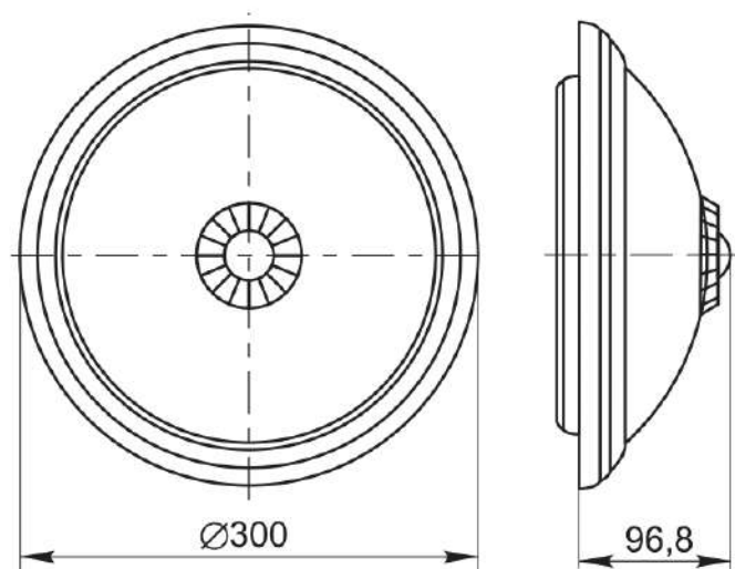
Рисунок 3 - НПО 3234Д
