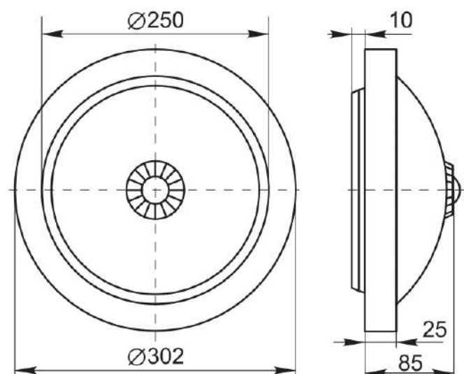
Рисунок 5 - НПО 3236Д
