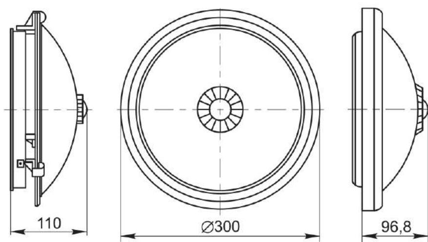
Рисунок 2 - НПО 3233Д
