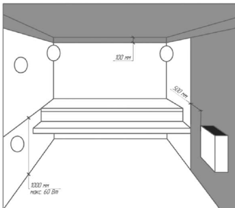
Рисунок 1 Установочные зоны светильника
