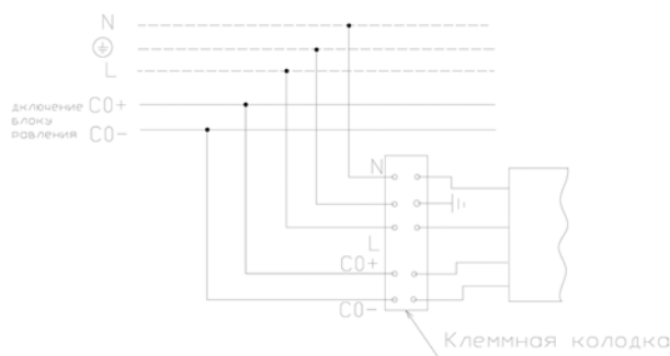
Схема подключения к питающей сети с регулируемым ЭПРА:
