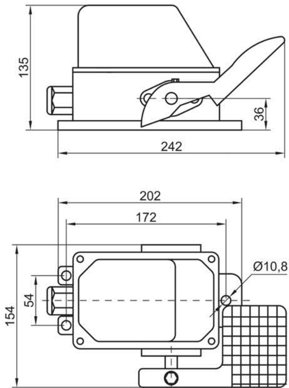
Рисунок 4. Габаритные и установочные размеры выключателей НВ-701 У1
