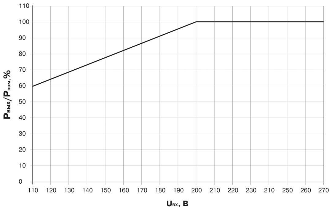
Рис 1. Зависимость выходной мощности от входного напряжения, где U_{\text{вх}} — входное напряжение, P_{\text{вых}} — выходная мощность, P_{\text{ном}} — номинальная (паспортная) выходная мощность
