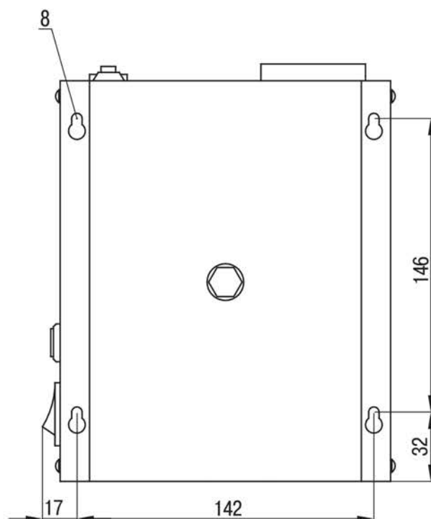
Рис 5. Задняя панель стабилизатора
