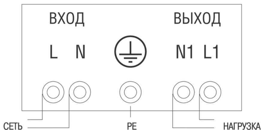
Рис 4. Схема подключения стабилизаторов
