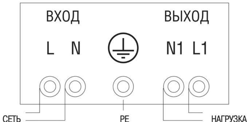
Рис 3. Схема подключения стабилизаторов от 3 до 12 кВА
