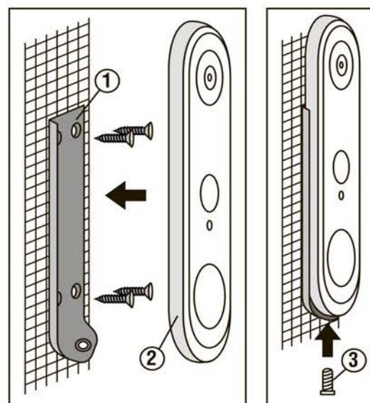
Рис. 1. Установка видеозвонка
