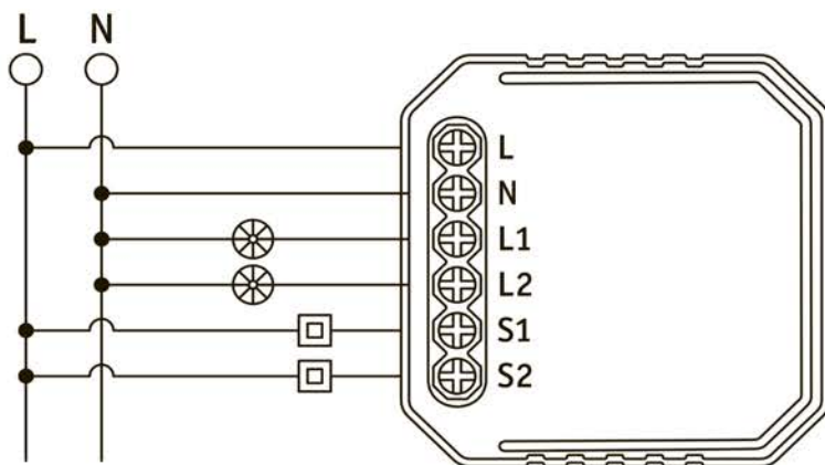
Схема подключения
