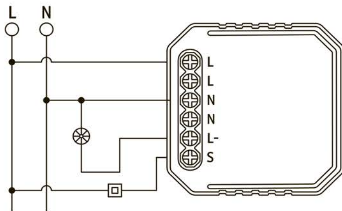
Схема подключения
