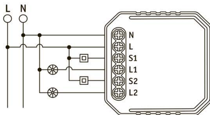
Схема подключения
