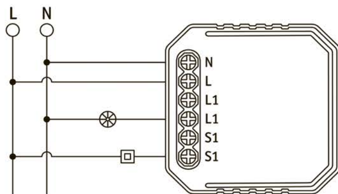
Схема подключения
