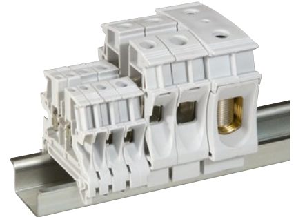
Единый профиль для клемм с шагом до 10 мм, одинаковая высота для клемм с шагом от 12 до 22 мм
