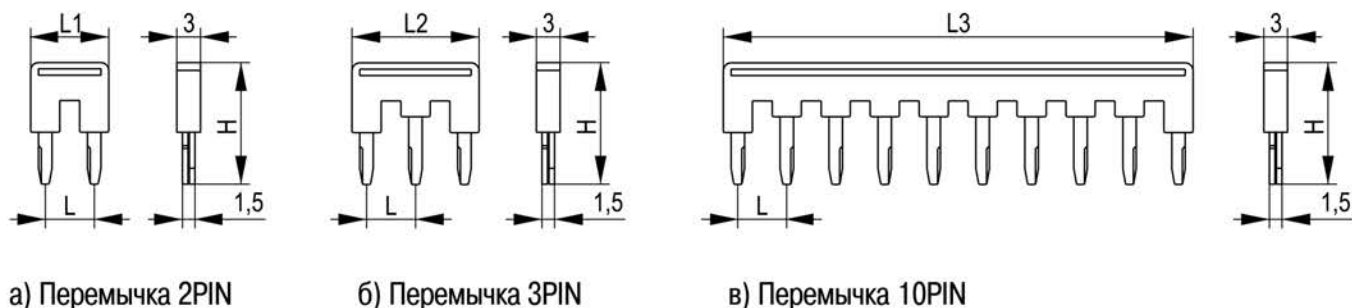
Рисунок 4 – Габаритные и установочные размеры перемычек для КПИ
