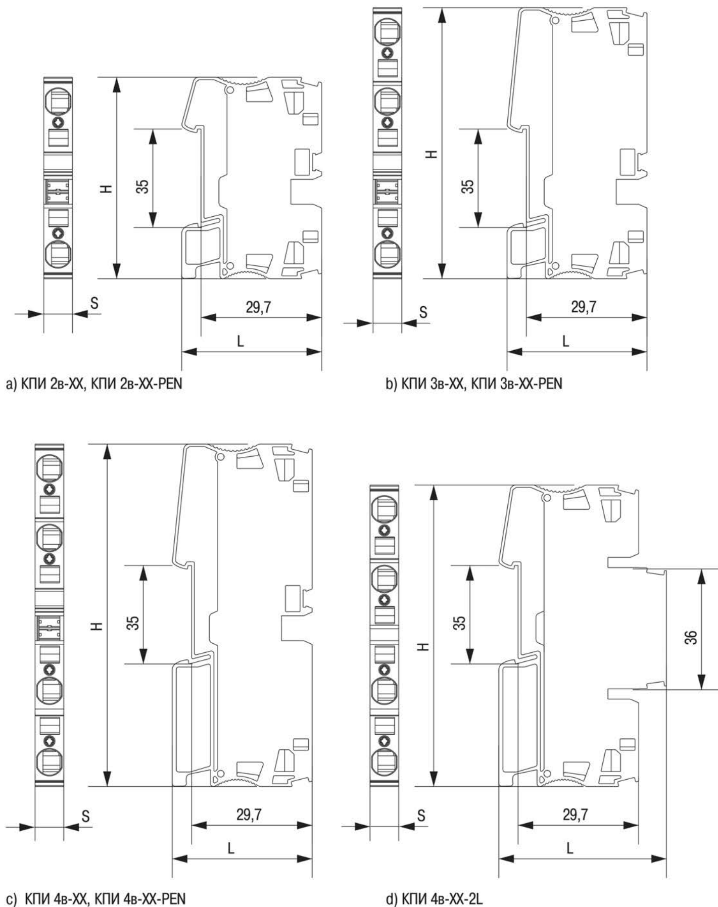
Рисунок 1 – Габаритные и установочные размеры клемм
