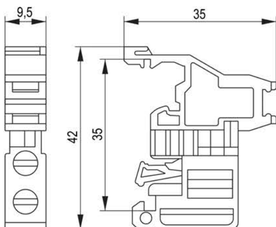
Рисунок 2 – Габаритные и установочные размеры стопора концевого
