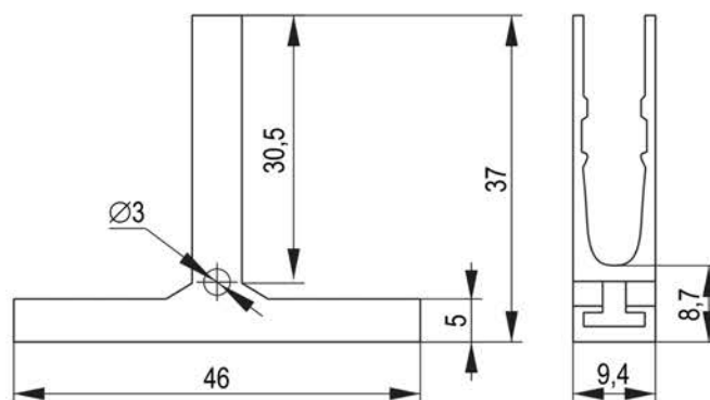
Рисунок 3 – Габаритные и установочные размеры держателя маркировки
