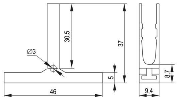
Рисунок 3 – Габаритные и установочные размеры держателя маркировки
