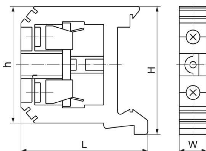
Рисунок 2 – ЗНИ для фазных проводников
