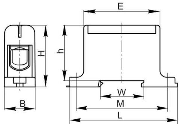
Рисунок 2 – КВС 16-95 (1/2), КВС 35-150
