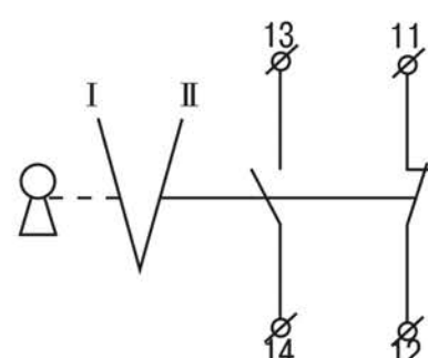
Рисунок 1 - Схемы электрические принципиальные переключателей LAY5 и дополнительных контактов к ним.
