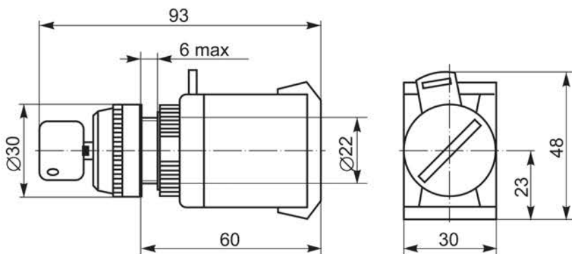
Переключатель AKS-22
