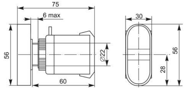
Кнопка APBB-22N
