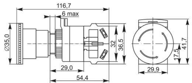
Кнопка D8-11MD
