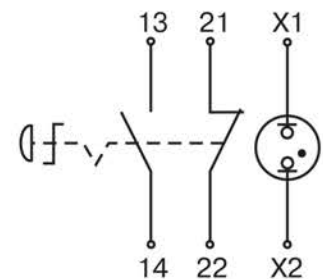
Кнопка ANE-22
