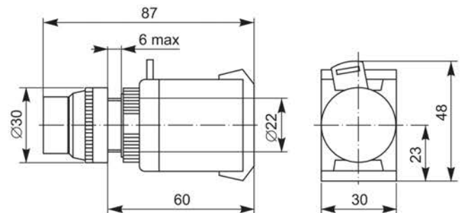
Кнопка ABLFP-22
