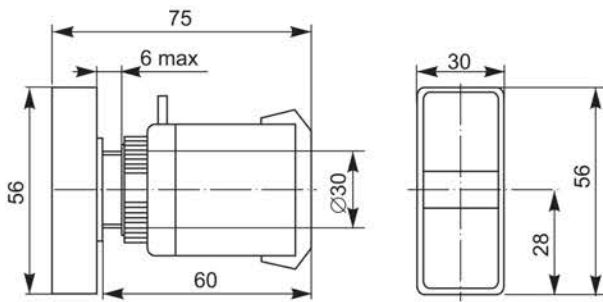
Кнопка PPBB-30N
