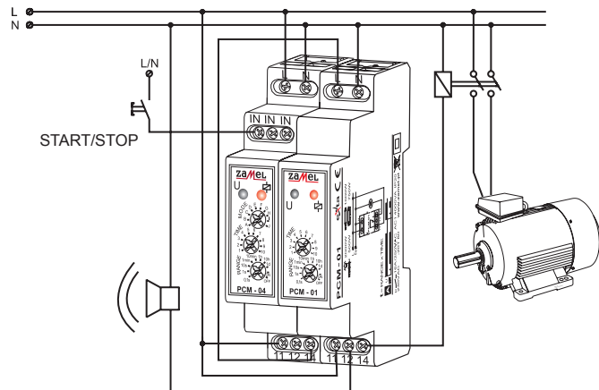
Система сигнализации перед включением двигателя (машины)
