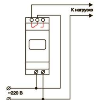
Схема подключения реле
