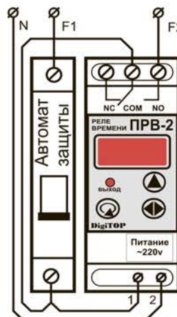
Монтажная схема подключения реле
