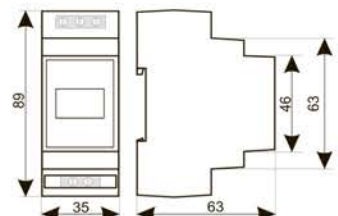
Габаритные размеры
