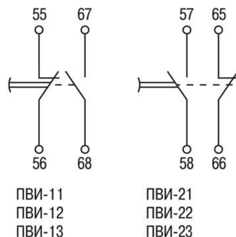
Рисунок 7 Электрические схемы ПВИ
