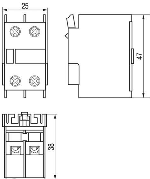
Рисунок 1 Габаритные размеры ПКИ-11, ПКИ-20
