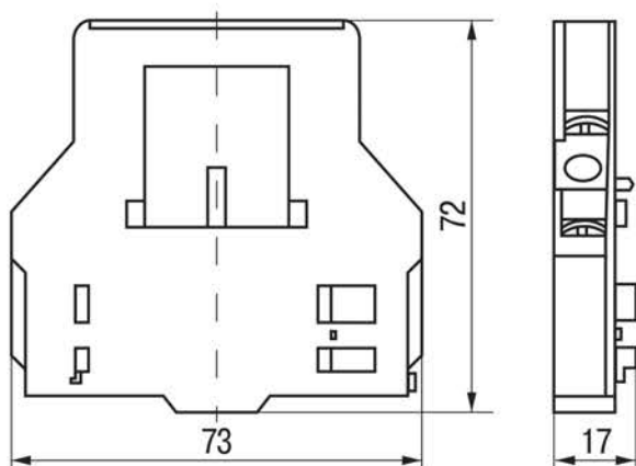
Рисунок 4. Габаритные размеры ПКБ
