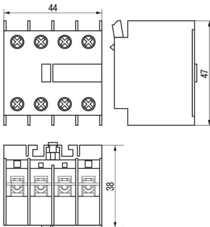
Рисунок 2 Габаритные размеры ПКИ-04, ПКИ-22, ПКИ-40
