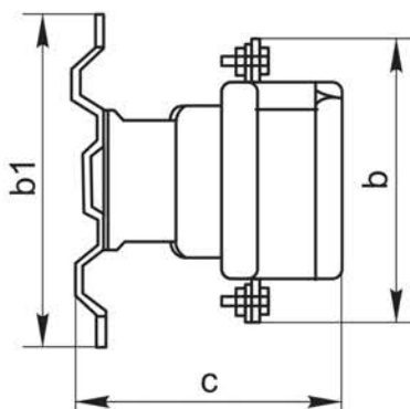
Рисунок 3 – КТИ-76303
