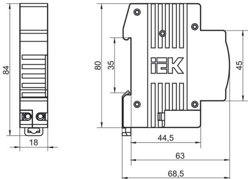
Рисунок 1 – Габаритные и установочные размеры устройства
