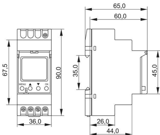
Рисунок 2 – Габаритные и установочные размеры таймера
