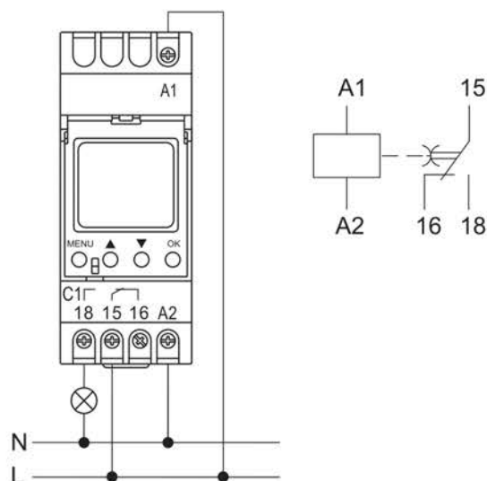
Рисунок 3 – Схема подключения таймера
