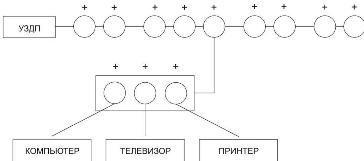
Рисунок 8 – Расширение зоны обслуживания удлинителем
