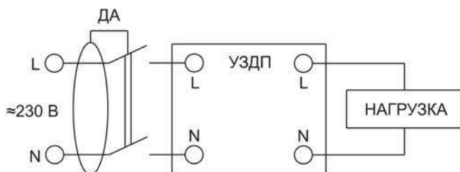
Рисунок 5 – Подключение устройства с дифференциальным автоматом (ДА)
