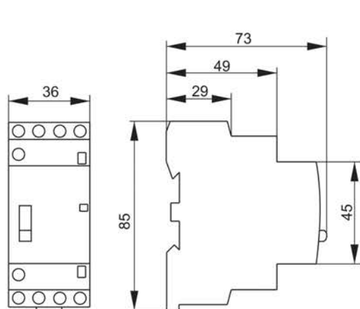
Контакторы KM20-22MP AC, KM25-22MP AC и KM20-40MP AC
