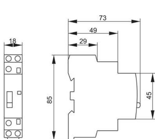
Контакторы KM20-20MP AC и KM20-11MP AC
