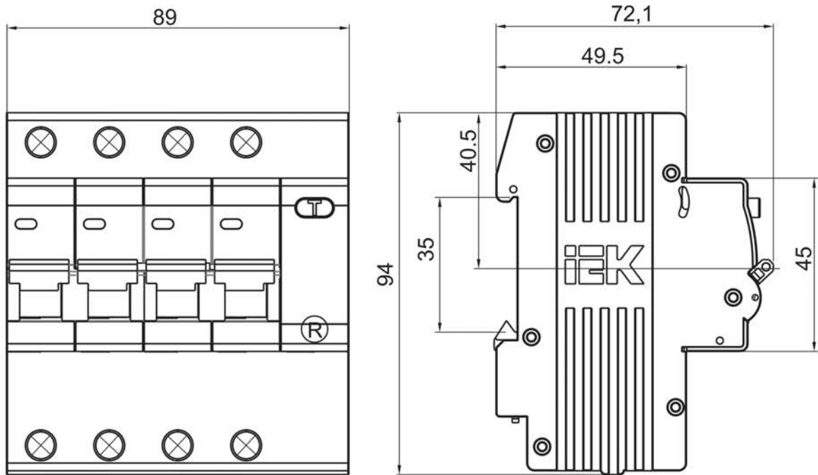
Рисунок 3 – Габаритные размеры АД14
