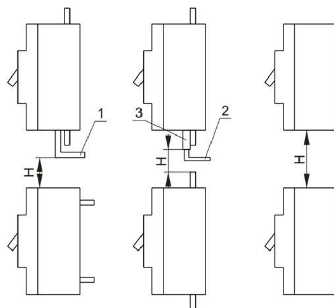
1 – Неизолированное присоединение; 2 – Изолированный кабель; 3 – Кабельные наконечники.
