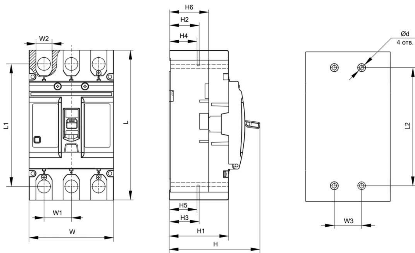
Рисунок 4 – Габаритные и установочные размеры выключателей
