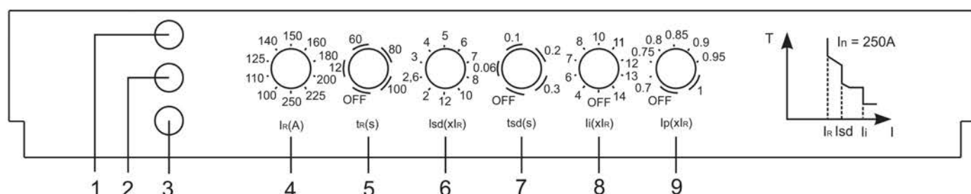
Рисунок 1 – Светодиоды и регуляторы выключателей (на примере BA88-35)
