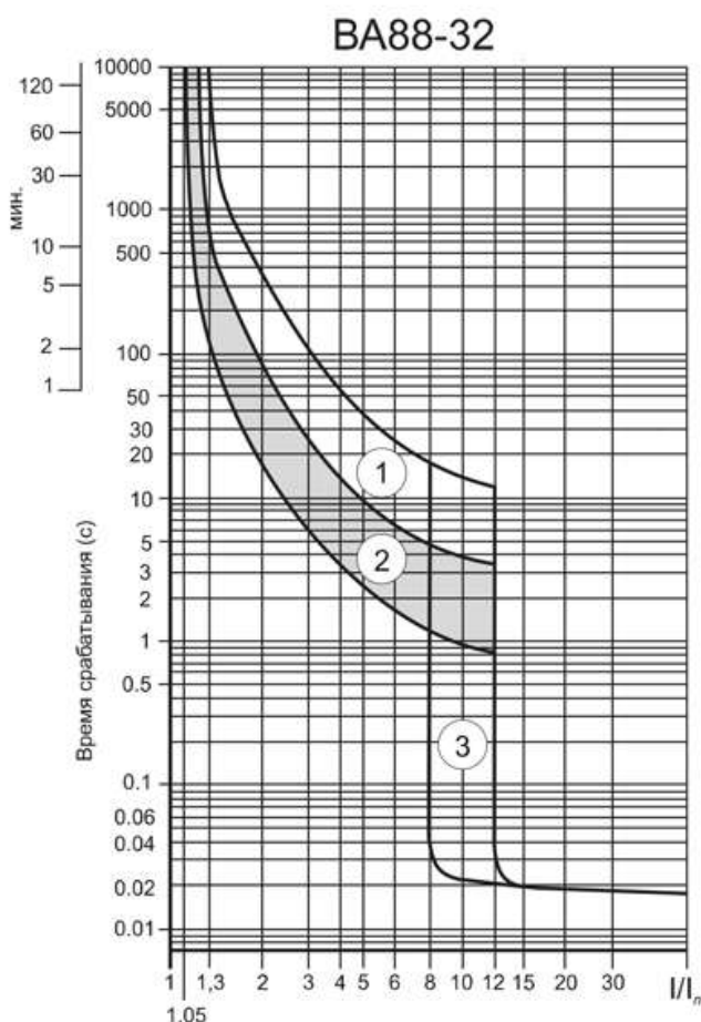
Рисунок 1 – Время-токовые характеристики выключателей BA88-32 и BA-33
