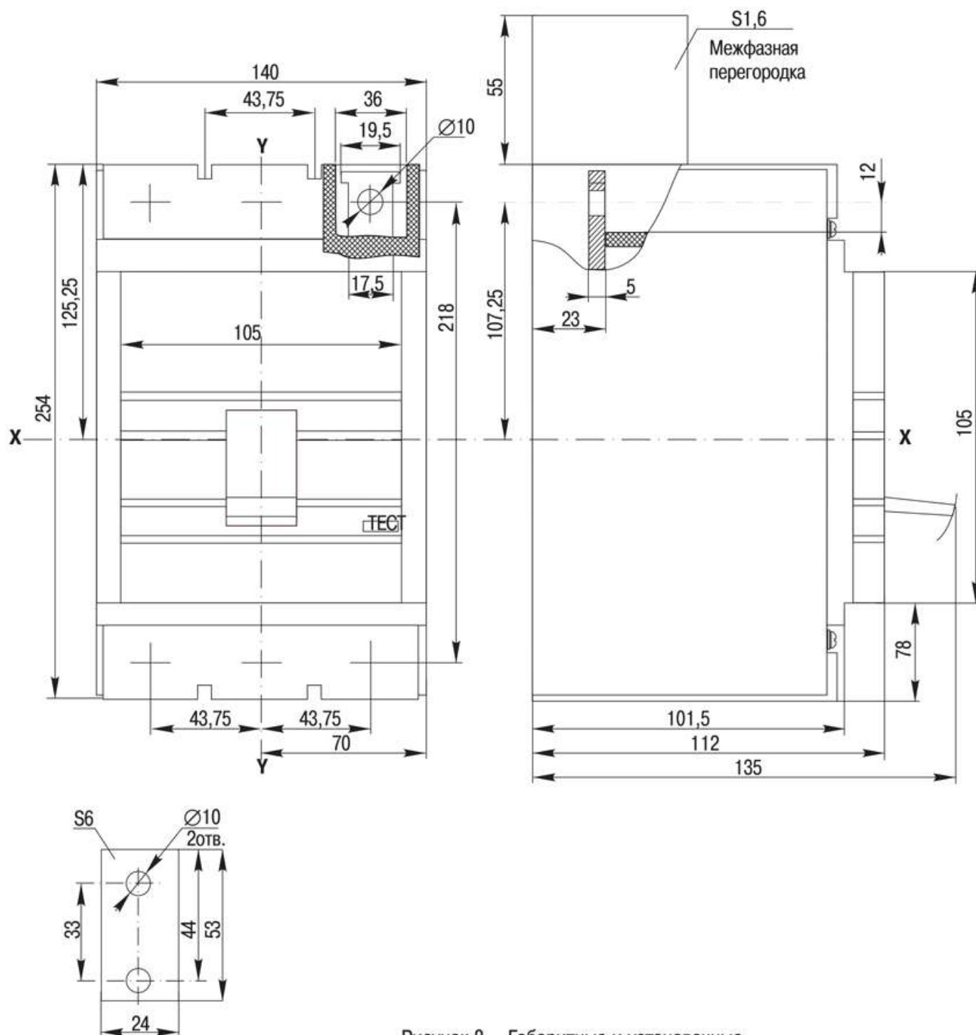
Наконечник-переходник
