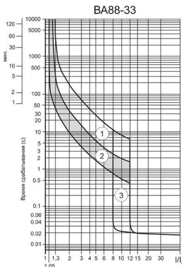
Рисунок 1 – Время-токовые характеристики выключателей BA88-32 и BA-33
