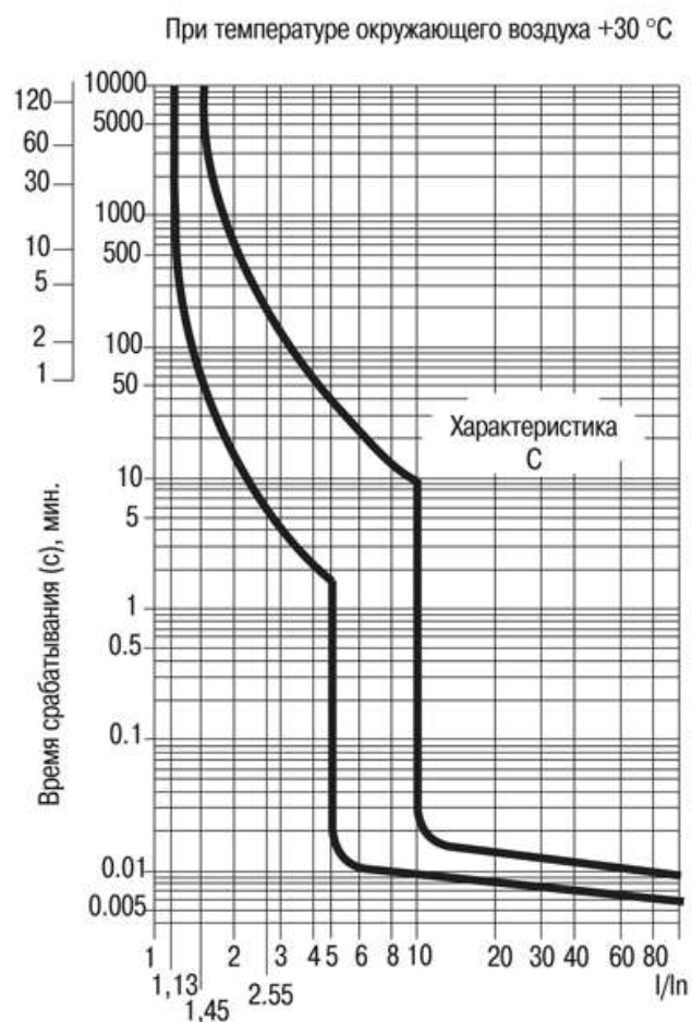
Рисунок 1 – Характеристика C
