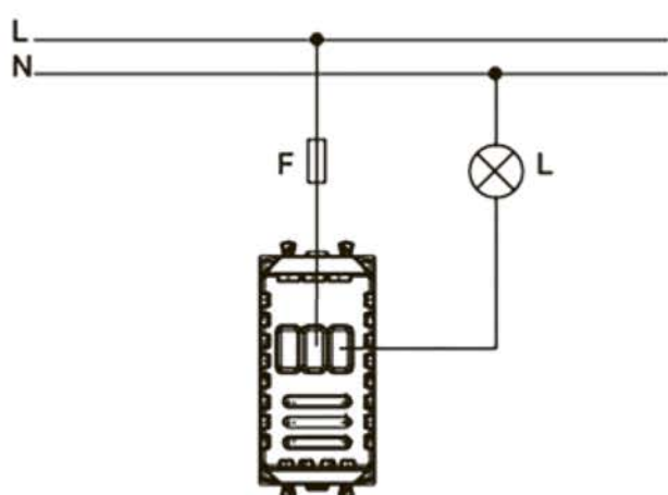
Схема 1. Совместное управление яркостью и включением лампы:
