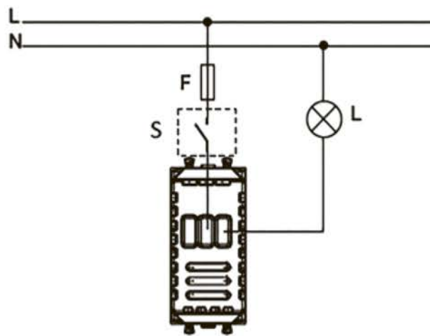
Схема 2. Раздельное управление яркостью лампы и ее включением:
