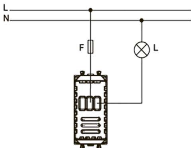
Схема 1. Совместное управление яркостью и включением лампы:
