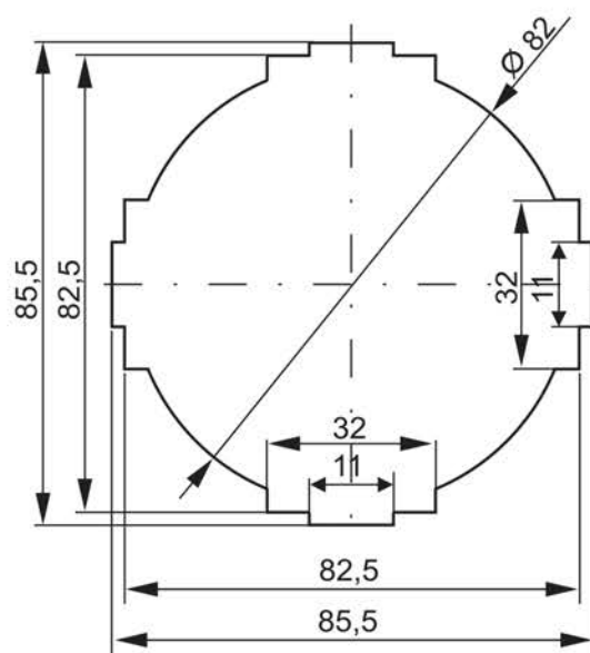
Рисунок 3 – Размеры отверстий под шины и кабели
