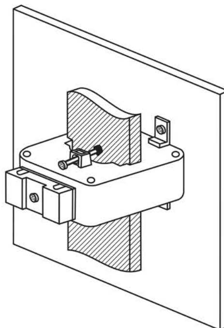
Рисунок 5 – Установка трансформаторов модификации ТТИ-85, ТТИ-100, ТТИ-125 на шине при помощи винтов
