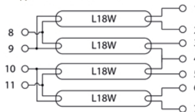
подключение 4 ламп 18Вт
