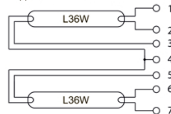
подключение 2 ламп 36Вт
