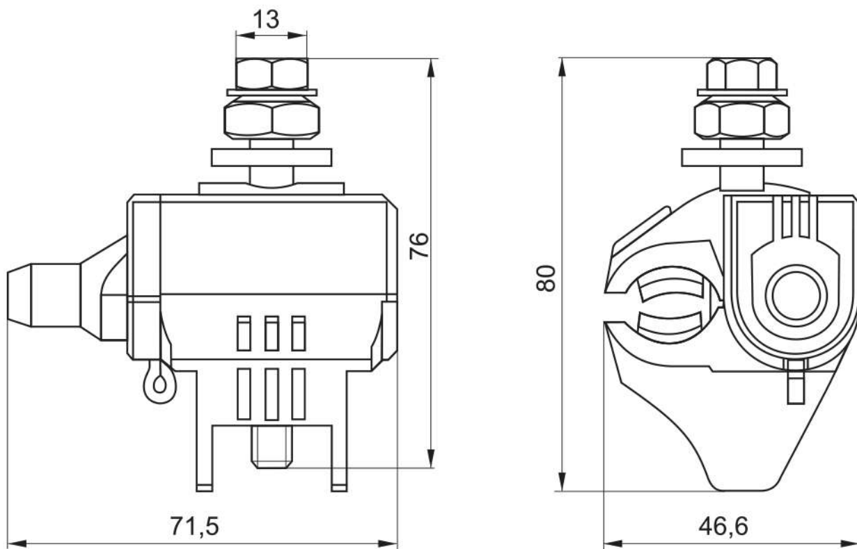
Рисунок 3. Зажим ЗСП35-95/6-35
