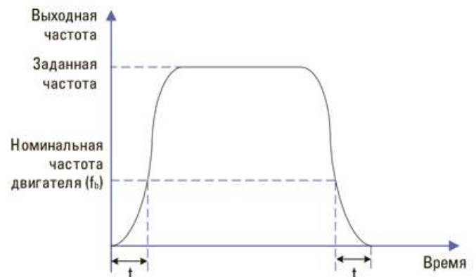
Картина В: схема S-кривой ускорения/торможения В
