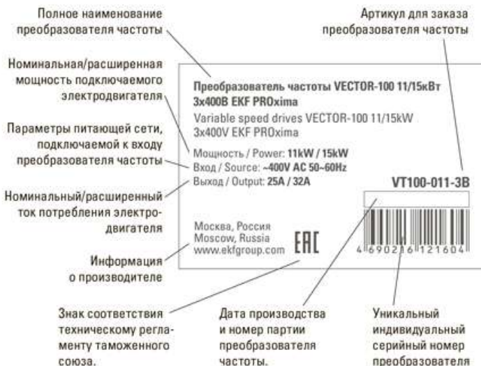
Рис. 2-2 Паспортная табличка.
