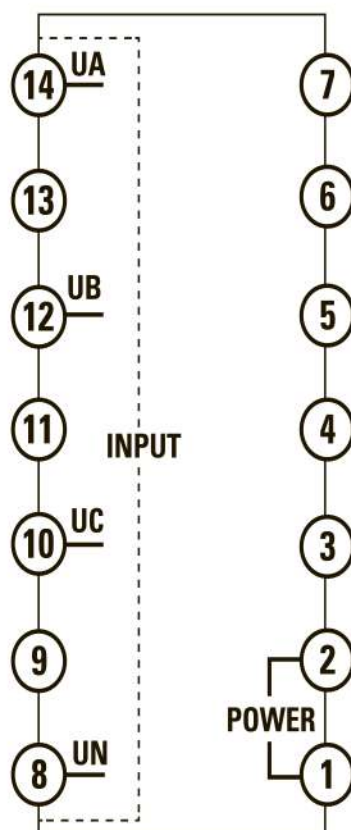
Рис. 7 Обозначение клемм для приборов размером 72x72
