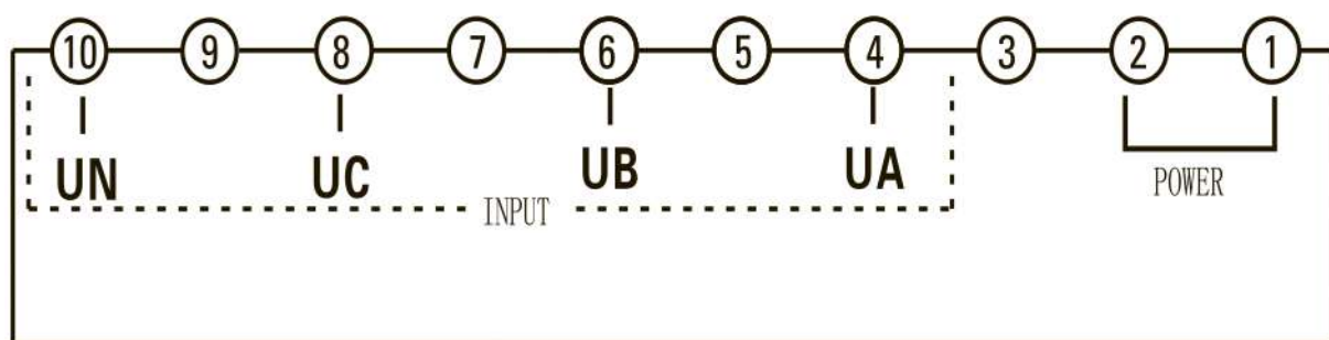
Рис. 6 Обозначение клемм для приборов размером 96х96
