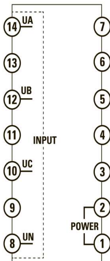
Рис. 7 Обозначение клемм для приборов размером 72х72
