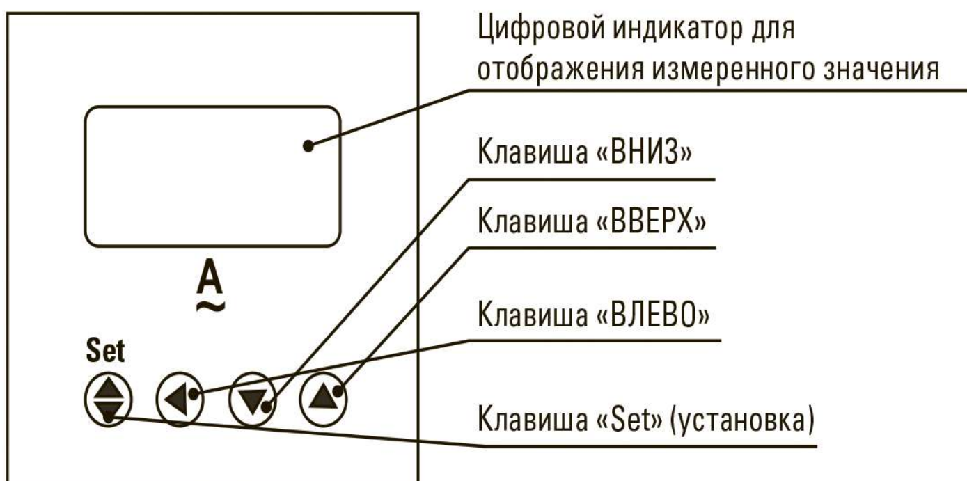
Рис.1 Лицевая панель прибора
